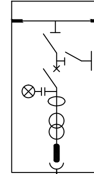
ŞEKİL-5 AKIM-GERİLİM ÖLÇÜ FONKSİYONEL BİRİMİ
